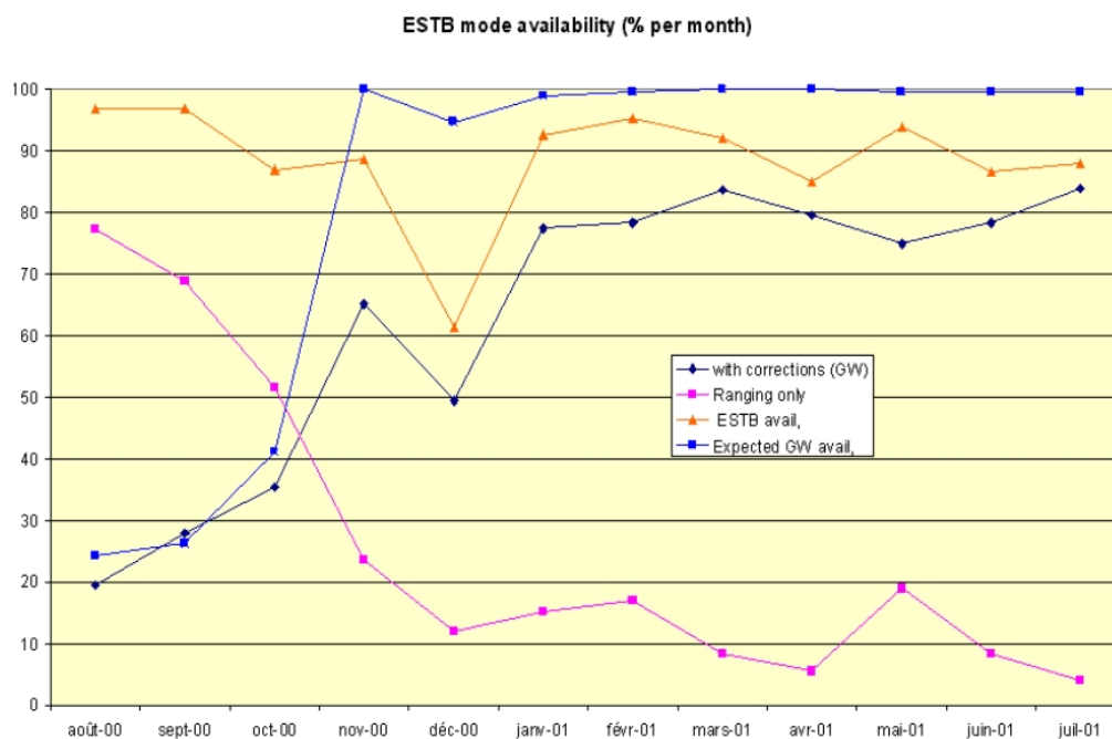
Fig. 2- ESTB SIS availability (% per month)
